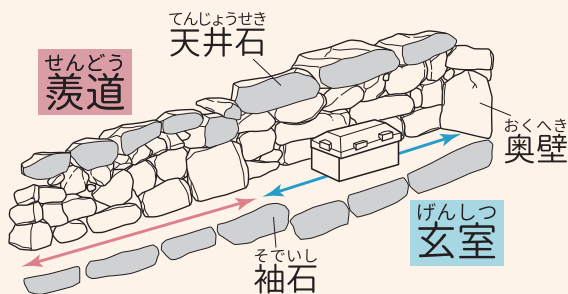
横穴式石室の構造と名称
